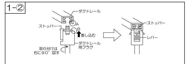
②ダクトレールへダクトレール用プラグを取り付けます。 A・Bの凹凸を合わせてダクトレール用プラグをダクトレールへ差し込み、プラグを右へ90°回して取り付けてください。 このとき、ストッパーがダクトレールに確実にハマっていることを確認してください。
