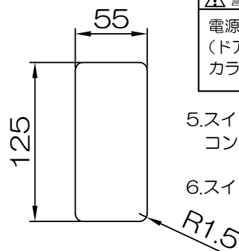
取付面開口穴寸法図
