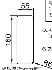
取付面開口穴寸法図
