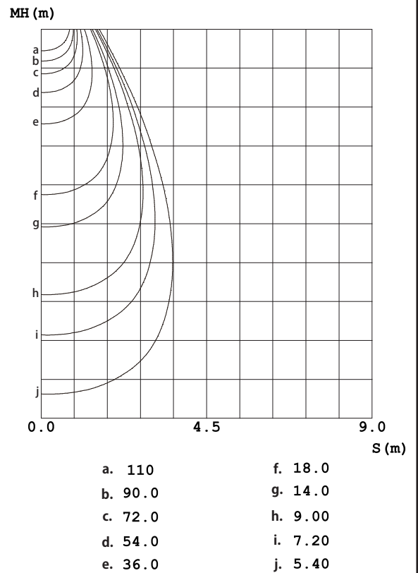
水平面照度
