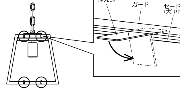
セード(小)取付側 押え部位置【図3】
