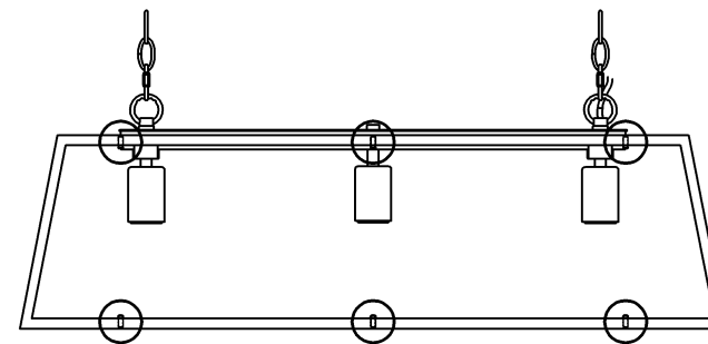
セード(大)取付側 押え部位置【図2】
