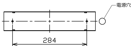
サポート取付寸法図
