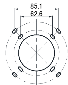
【取付寸法図】
