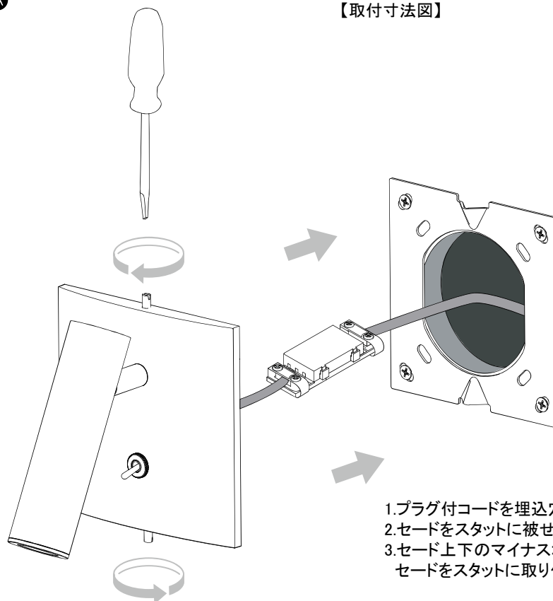
【取付寸法図】
